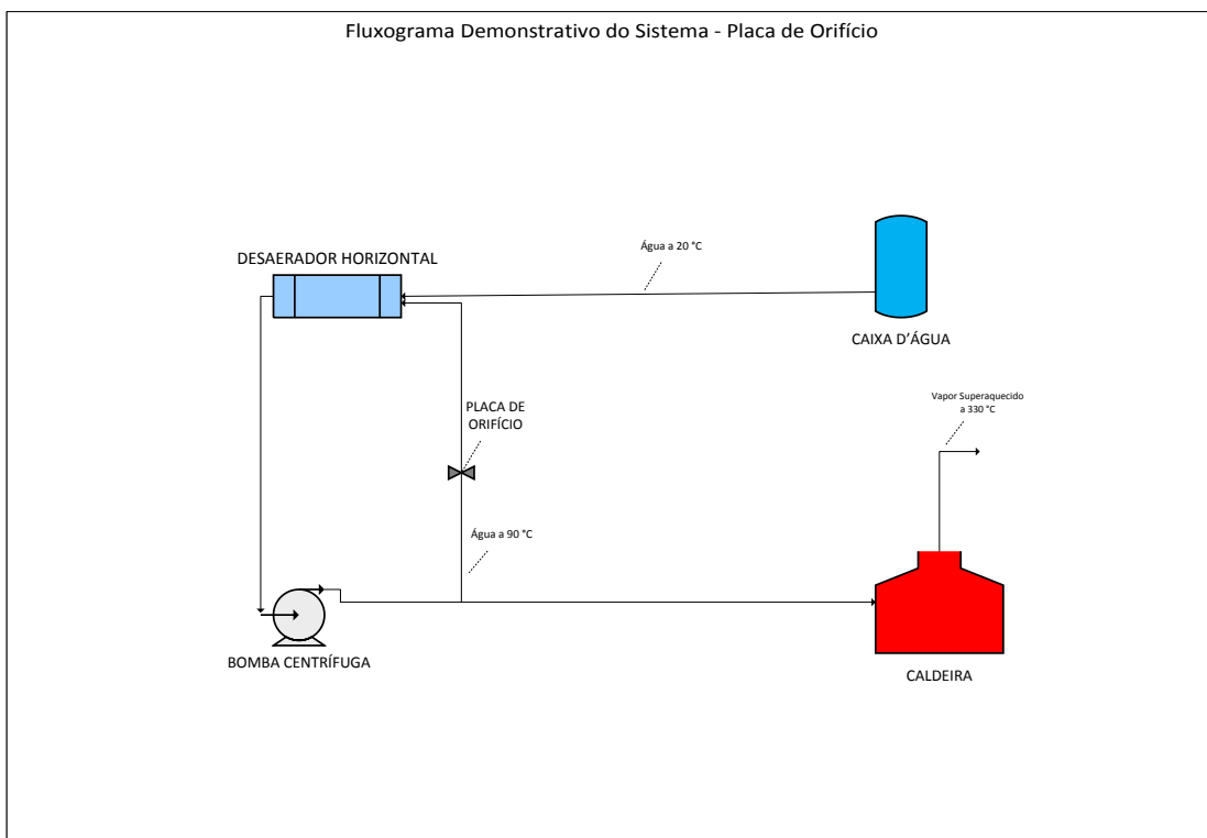
FIGURA 4 – Fluxograma do Sistema – Placa de Orifício
