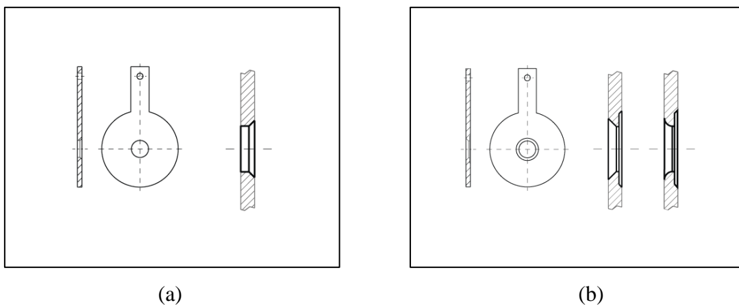
FIGURA 1 – Modelos de placas de orifício
