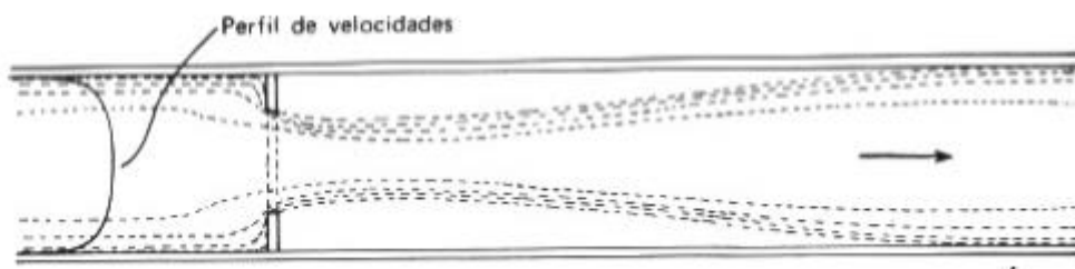
FIGURA 2 – Perfil de escoamento ao passar por uma placa de orifício
